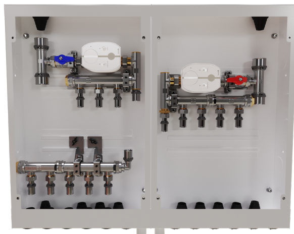
Eksempelskap med parkobling
