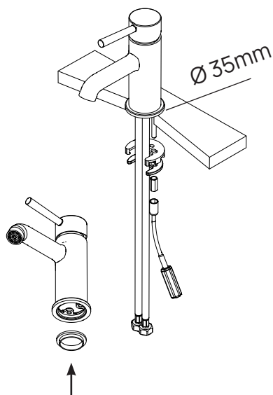
Montering med base plate
