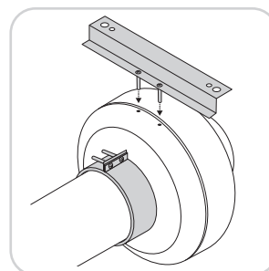
Montering med monteringsklämma och -beslag (tillbehör).
