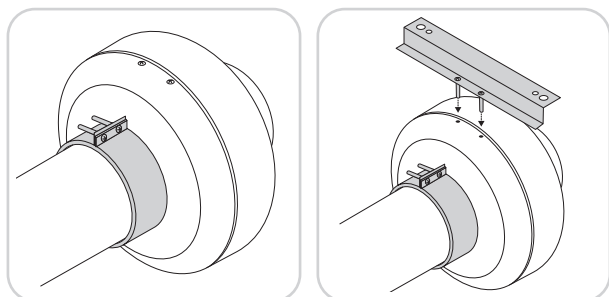
Asentaminen käyttäen asennussankaa ja -kiinnikettä (lisävaruste).
