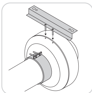
Montering med monteringsklemme og – brakett (tilbehør).
