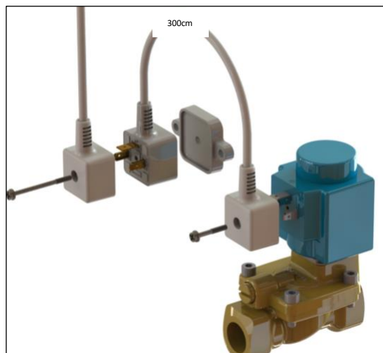
På denne illustrasjonen framstår skjøtekabelen kort, den reelle lengden 300cm.
